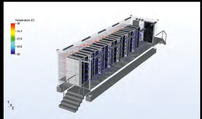
Luftstromlinien in einem nicht redundanten Gehäuse ohne Kaltgangeinhausung.
